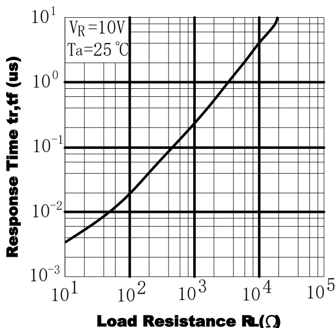
图.5 响应时间与负载电阻
