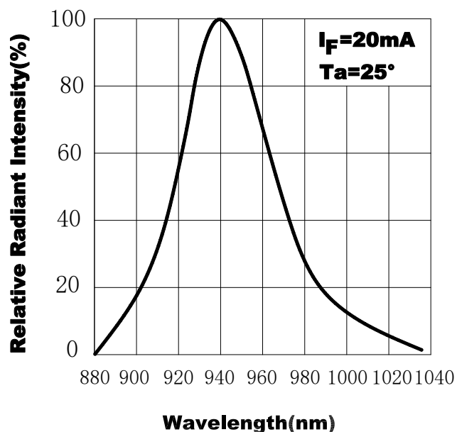
图.2 频谱分布
