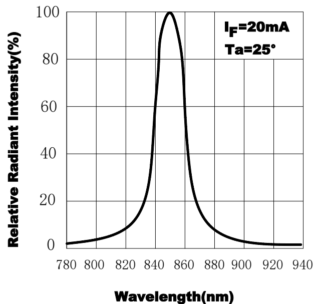
图.2 频谱分布
