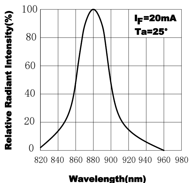
图.2 频谱分布
